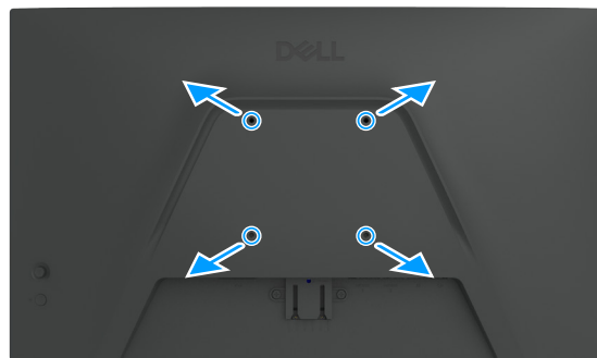
Afbeelding 18. VESA-wandbevestiging (optioneel)
