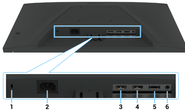
Afbeelding 3. Onderaanzicht
